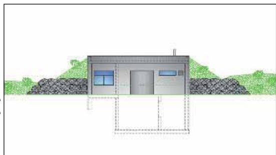
Das neue Filterbauwerk für die Wasseraufbereitung wird unterhalb des Hochbehälters Rietz errichtet
